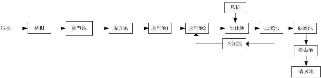
图 5.3-1 服务设施污水处理工艺流程框图
