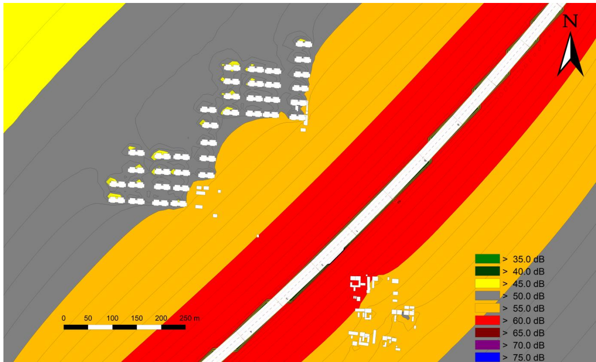
图 4.2-8 运营中期典型路段等声级线示意图（昼间）
