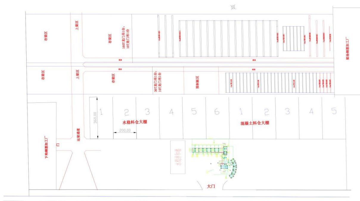
图 2.1-8 综合场站平面布置图
