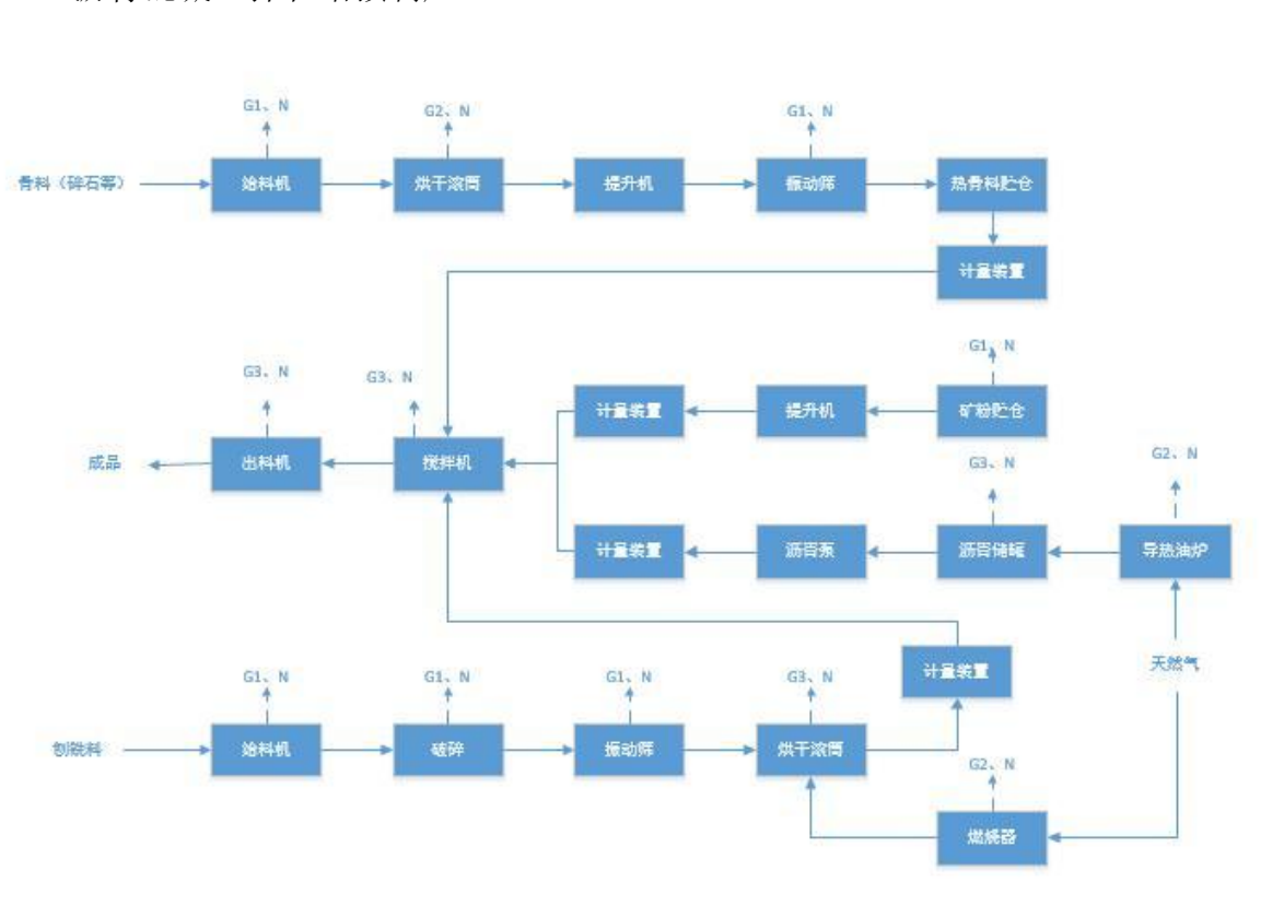
图 2.2-7 项目沥青混凝土拌和站工艺流程及产污节点图
