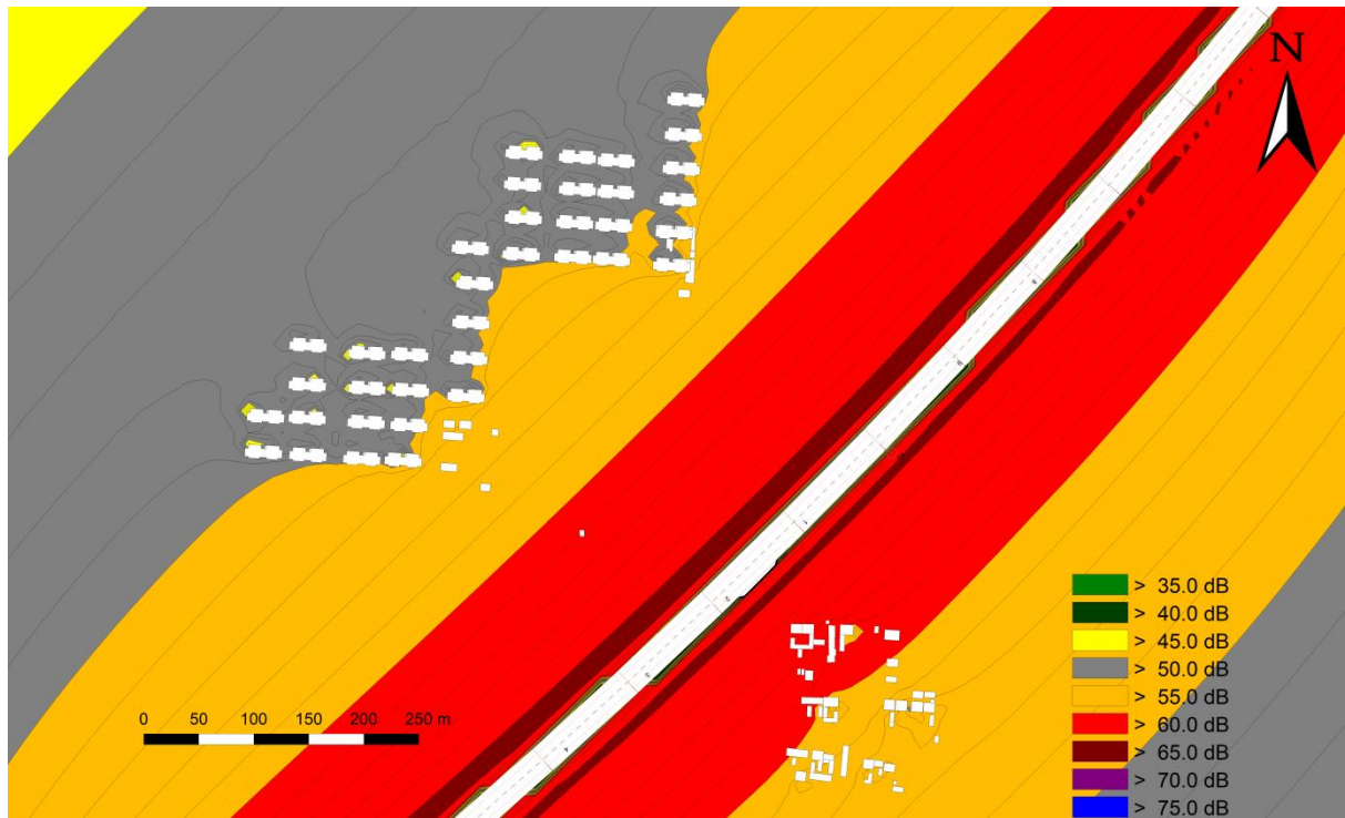
图 4.2-10 运营远期典型路段等声级线示意图（昼间）
