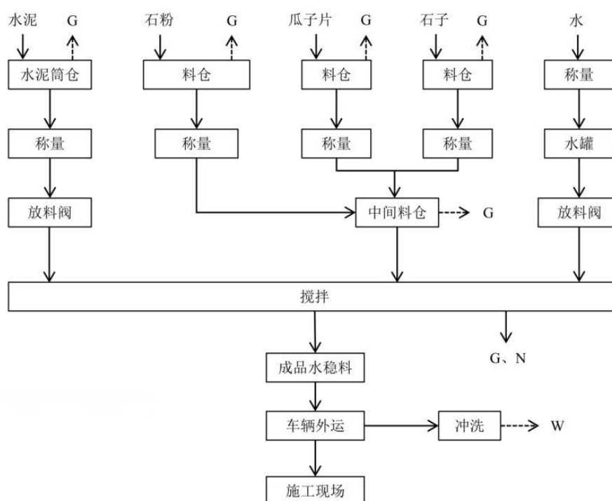
图 2.2-3 水稳拌和站生产工艺流程及产污节点图
