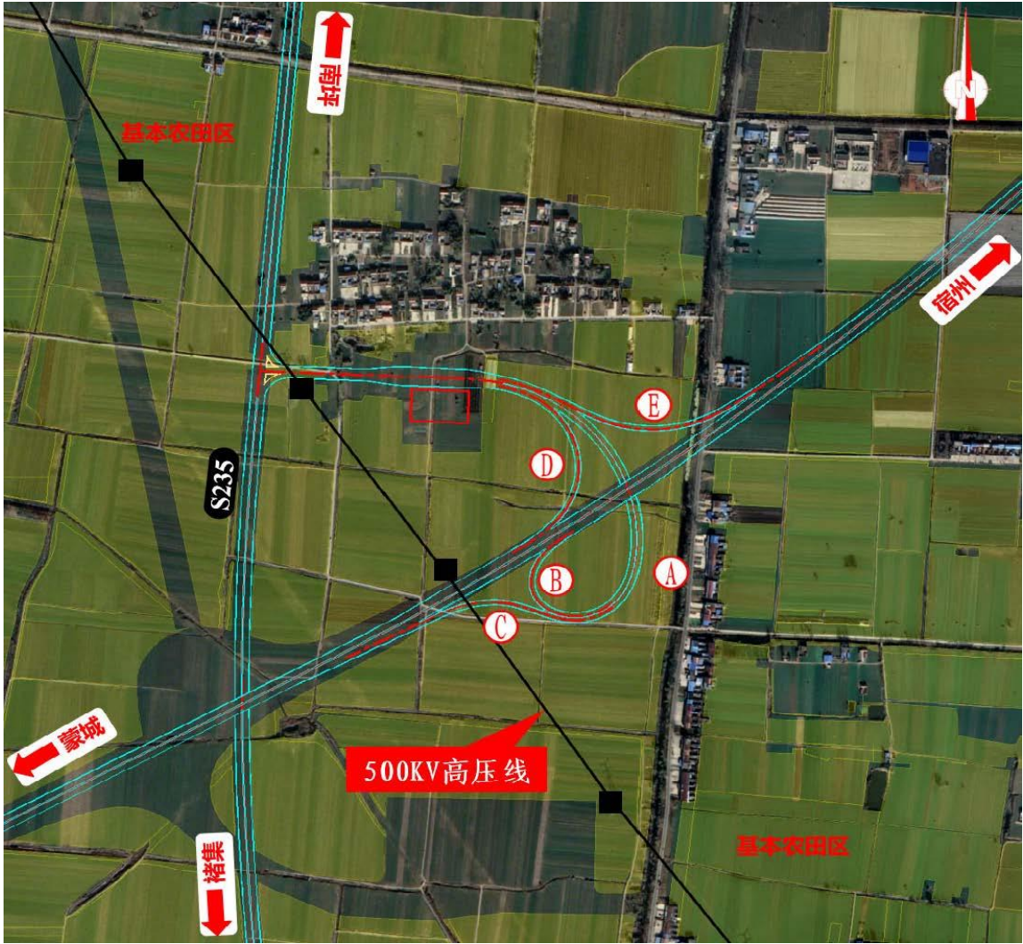
图 2.1-6 双堆集南互通平面布置示意图
