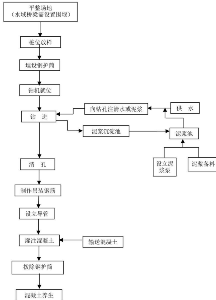
图 2.1-12 桥梁基础施工工艺示意图
