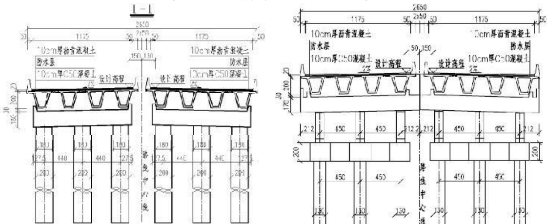
图 2.1-5 解河大桥断面布置图
