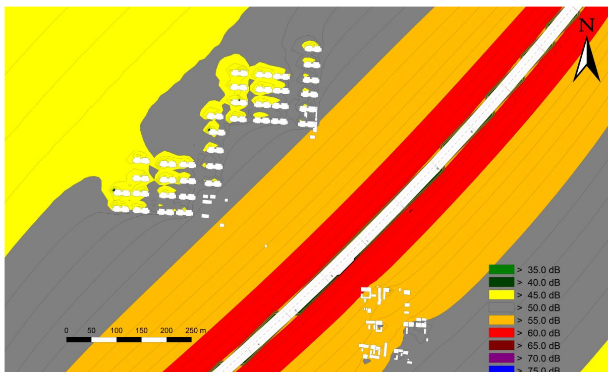
图 4.2-6 运营近期典型路段等声级线示意图（昼间）
