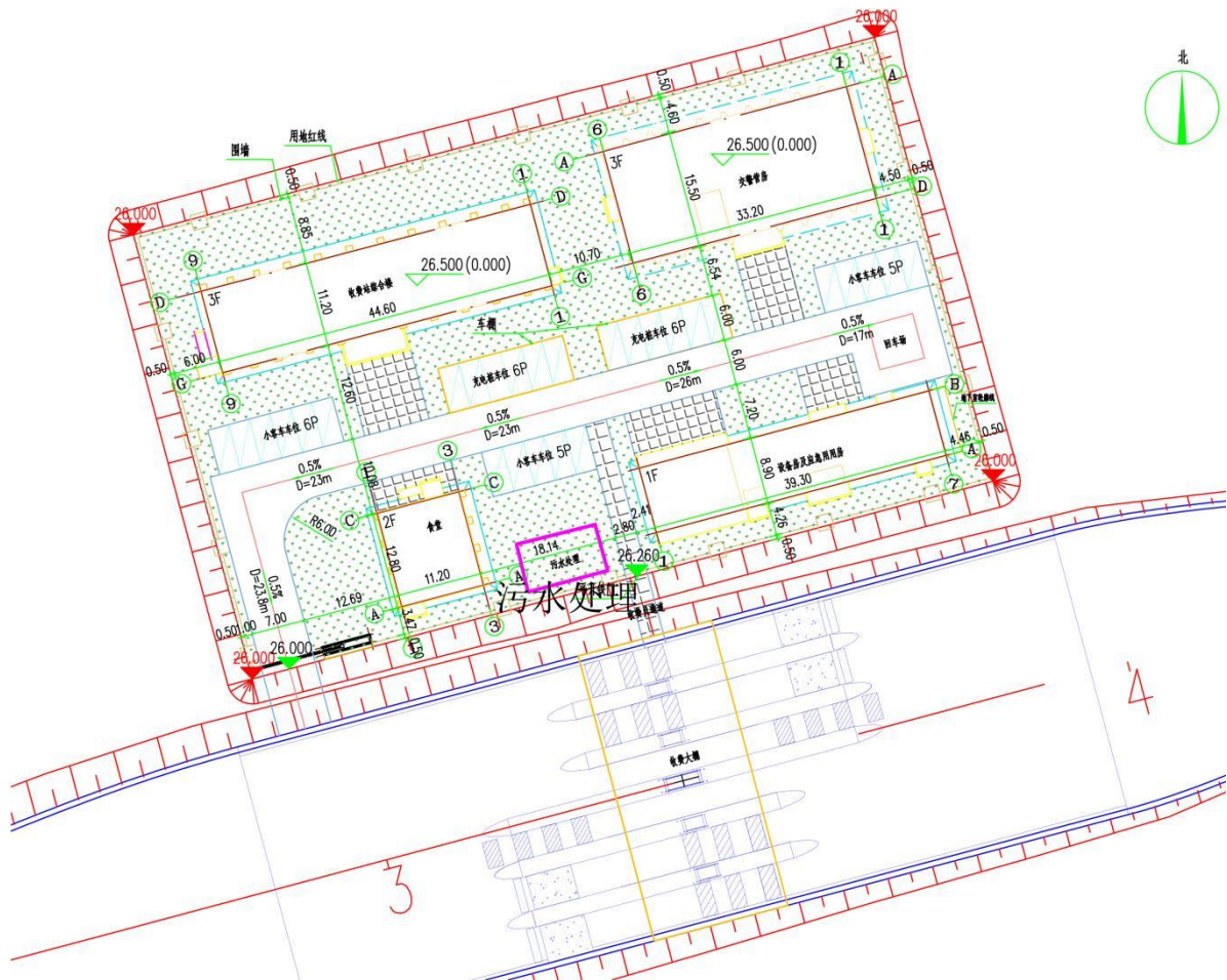
图 2.1-7 双堆集南收费站总平布置图
