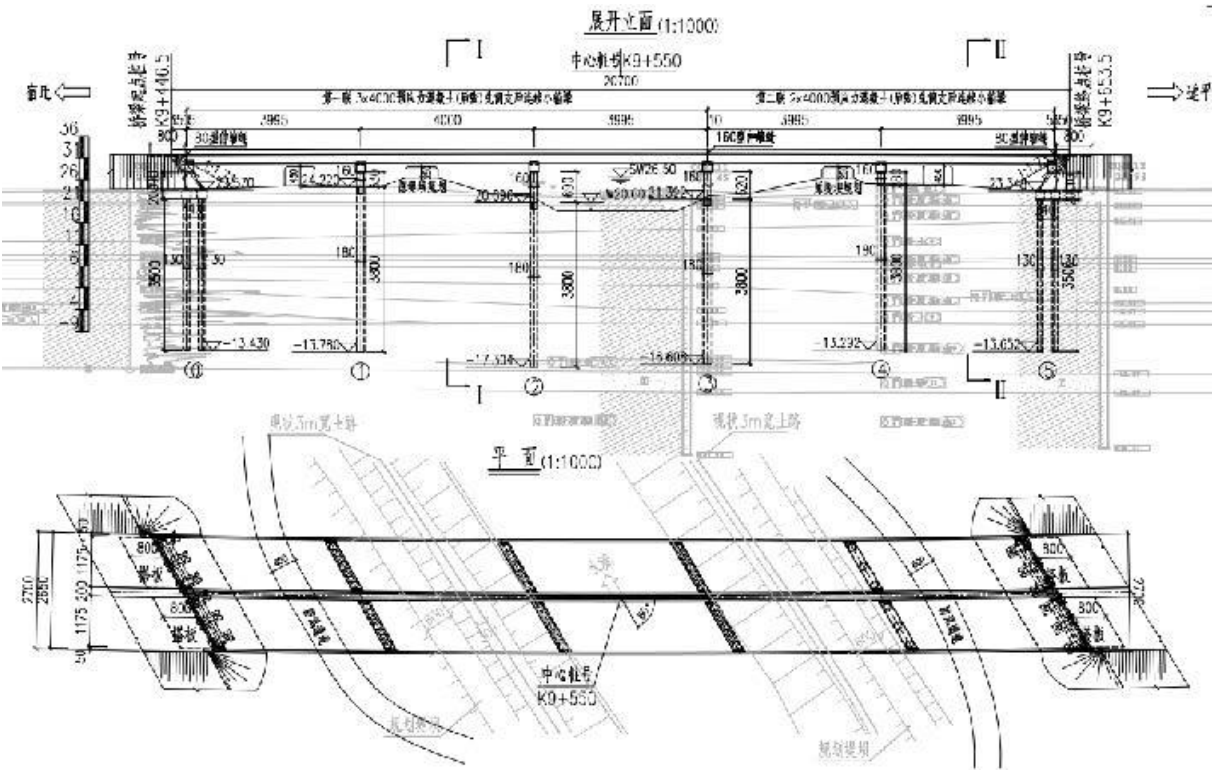
图 2.1-4 解河大桥桥型布置图
