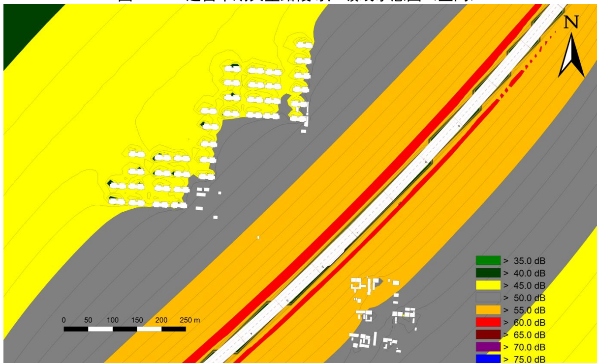
图 4.2-9 运营中期典型路段等声级线示意图（夜间）
