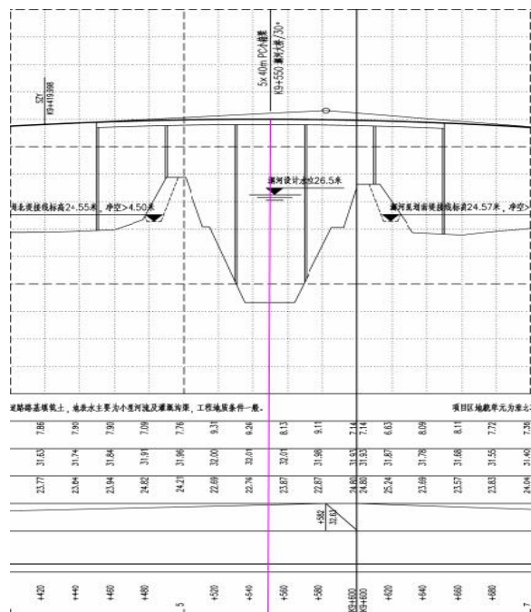
图 5.3-2 解河大桥路段局部纵断面示意图
