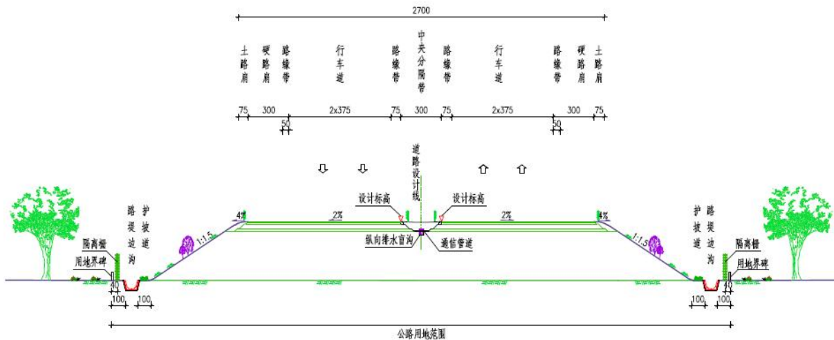
图 2.1-2 路基标准横断面布置示意图
